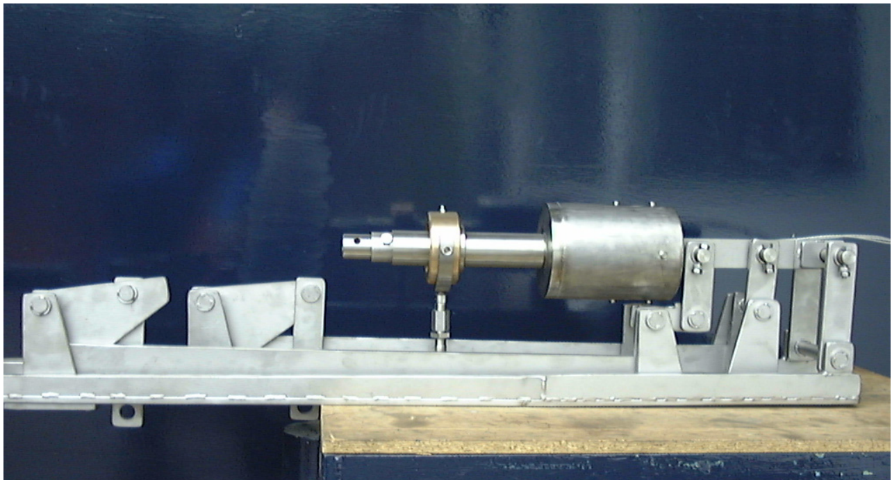
Abbildung: Gleitlagerprüfvorrichtung mit axialer und radialer Belastungsmöglichkeit
